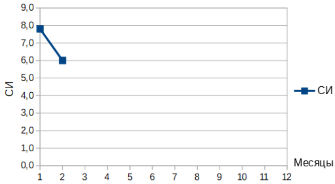
Рис. 8 — Годовой ход СИ и НП
