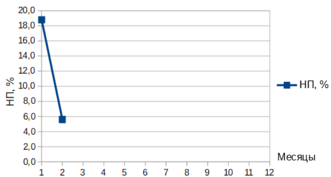
Рис. 20 — Годовой ход СИ и НП
